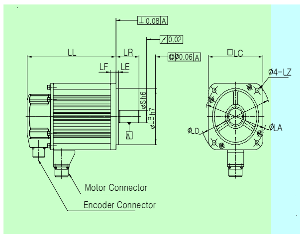
Motor connector (MS 3102A~)
